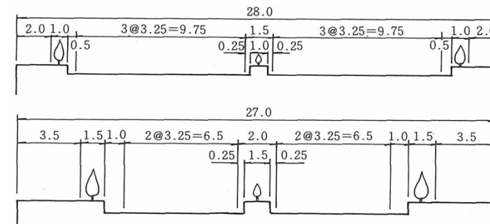
改築後
